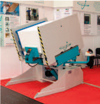
Innovation: der neue Stapelwender RD1000 PA-I/R+S mit Ionisierung und vollautomatischen Seitenarmen.
